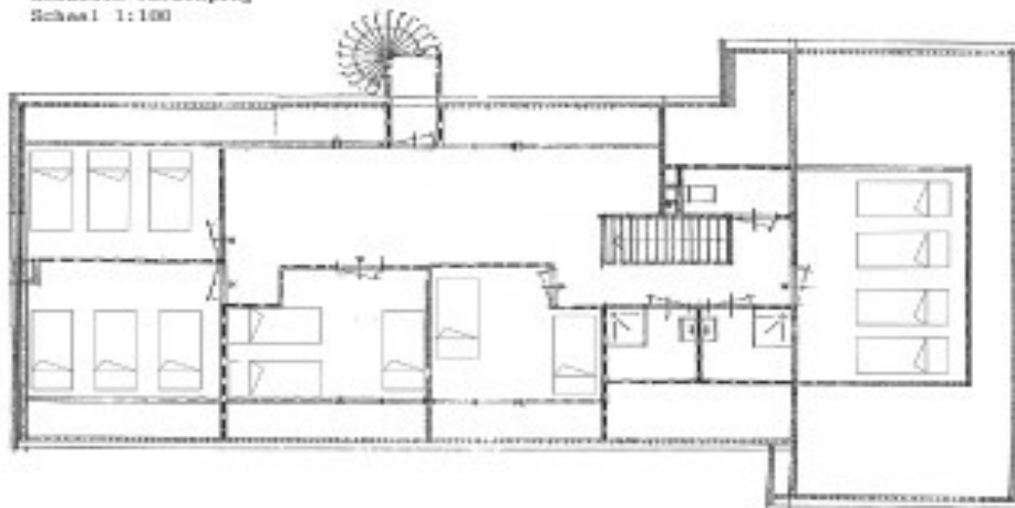
Landhuis verdieping Schaal 1:100
