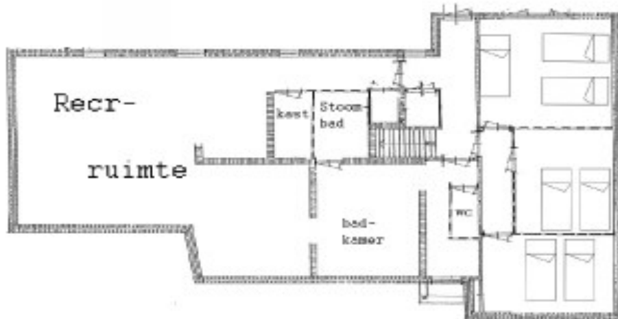
Landhuis souterraine Schaal 1:100
